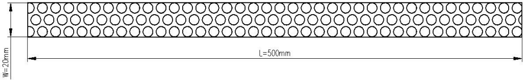
图 1 折式滤筒展开尺寸示意图
