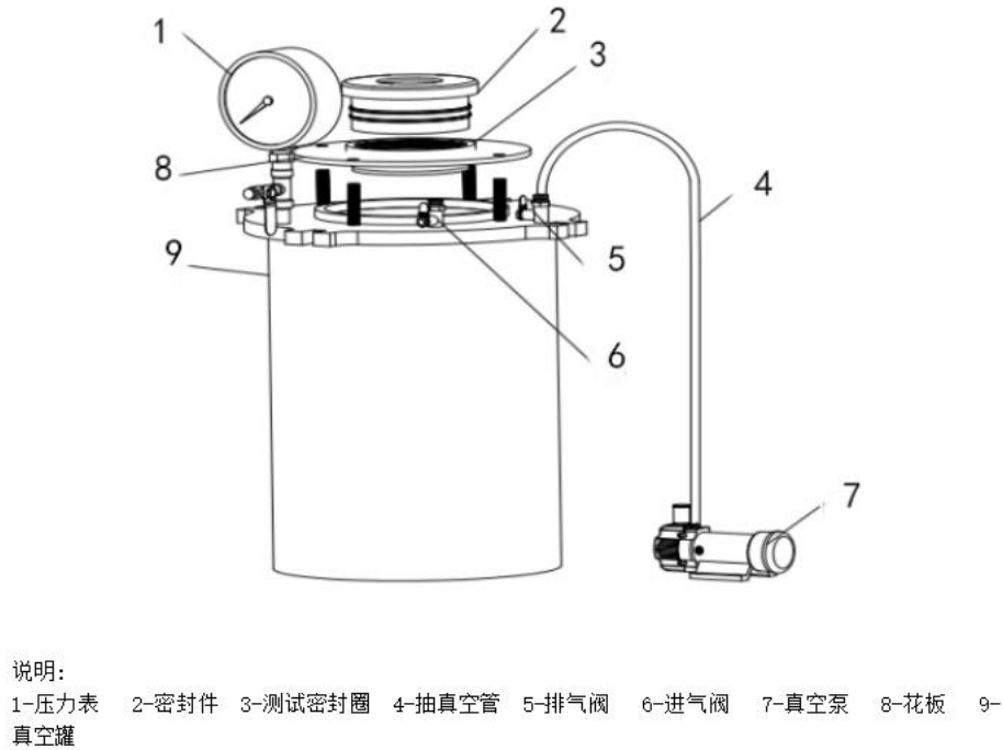
图 D.1 密封性能测试仪示意图
